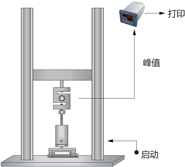
测力机
