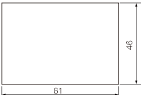
开孔尺寸
