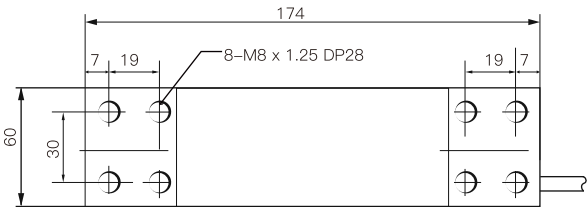
俯视图
