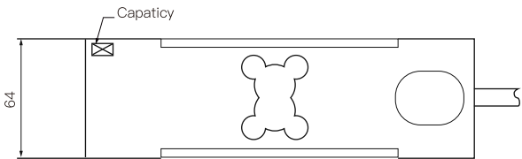
主视图
