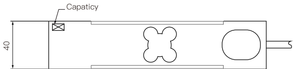
主视图
