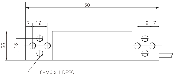
俯视图
