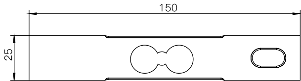
主视图
