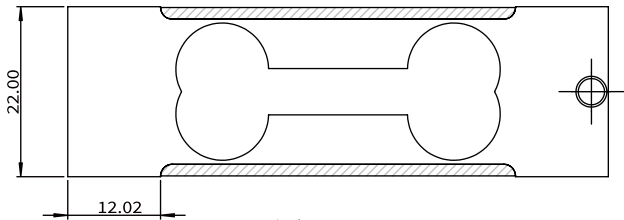
主视图
