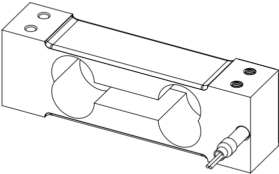
主视图
