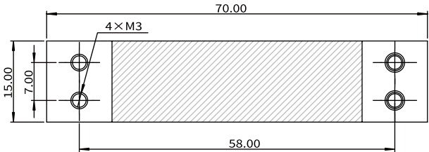
俯视图
