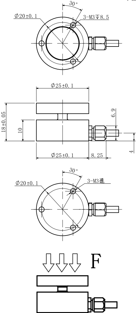
受力示意
