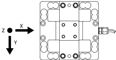
受力方式 ▲ Load Direction
